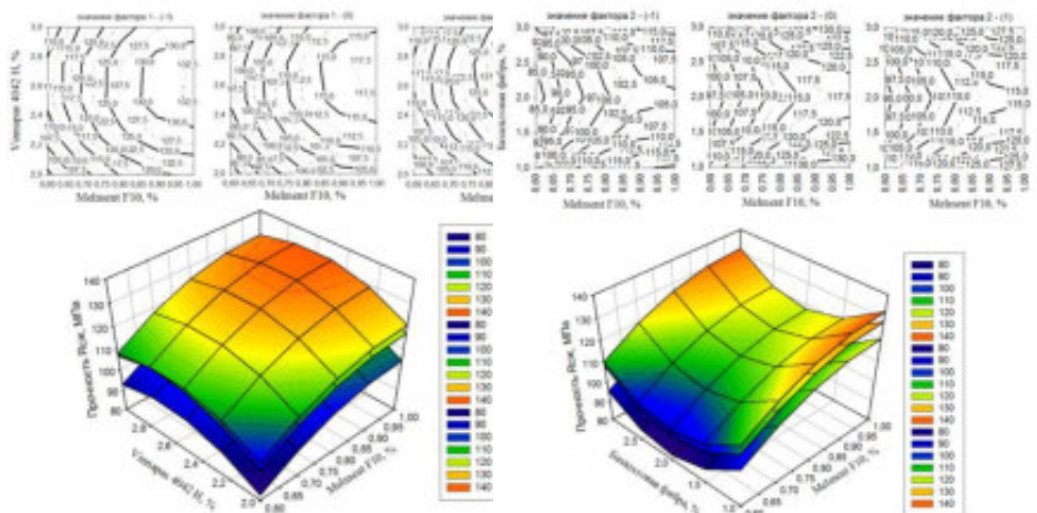
Рисунок 1 – Номограммы зависимости прочности затвердевшего состава от концентрации Melment F10 и Vinnapas LL 4042 H
