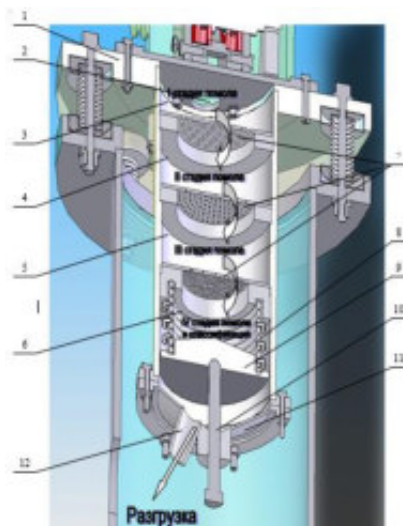
Рисунок 2 - Принципиальная схема работы мельницы
