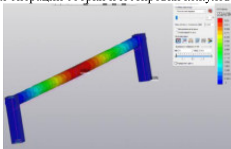
Рисунок 2 - Зоны повышенных напряжений в области крепления поворотной оси
