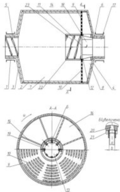
Рисунок 1. - Шаровая мельница с разгрузочным устройством:
