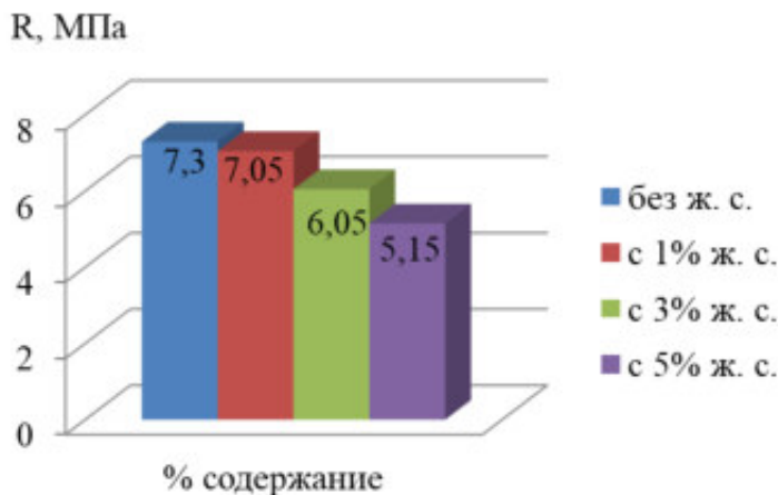
Рисунок 3 - Прочностные характеристики образцов в зависимости от содержания жидкого стекла
