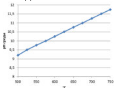
Рисунок 1 - Зависимость pH водной вытяжки от температуры обжига.
