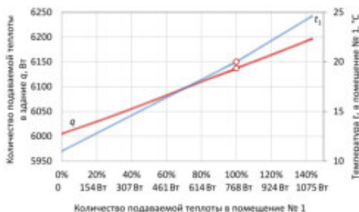
Рисунок 3 - Общий расход теплоты для здания и температура в помещении № 1 при изменении количества теплоты, подаваемого в помещение № 1, и поддержания температуры 20°C в остальных
