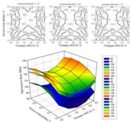
Рисунок 3 – Номограммы зависимости прочности затвердевшего состава от концентрации Vinnapas LL 4042H и базальтовой фибры
