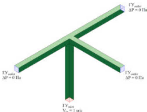
Рисунок 1 - Компьютерная модель равносторонней крестовины с заданными входным и выходными граничными условиями
