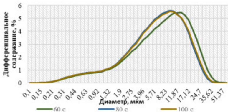
Рисунок 3 – Зависимость распределения частиц по размерам от времени помолы ОТМ
