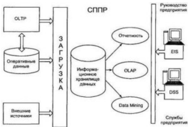
Рисунок 2 - Архитектура системы поддержки принятия решения
