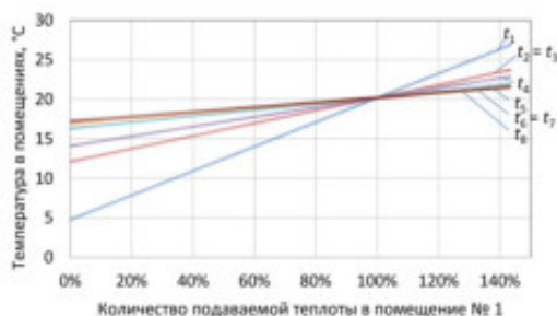
Рисунок 1 - Температура в помещении при изменении количества теплоты, подаваемого в помещение № 1
