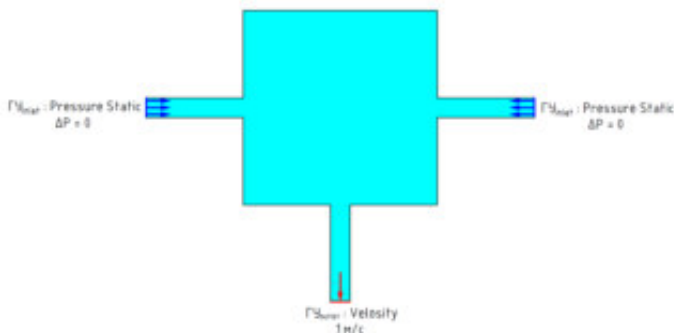
Рисунок 1 - Область проектирования и граничные условия задачи
