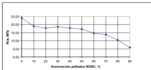
Рисунок 3 - Влияние добавок ЖСБС на прочность Г-5
