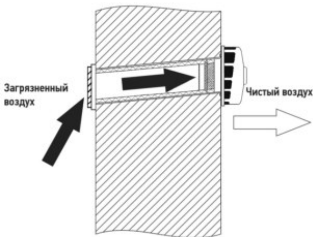
Рисунок 1 - Схема стенового приточного клапана
