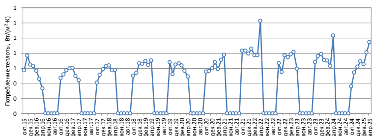
Рисунок 5 - Удельный расход тепловой энергии по месяцам
