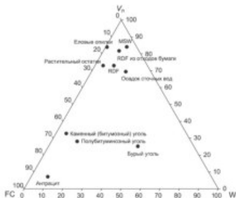
Рисунок 1 - Тройная фазовая диаграмма содержания летучих веществ, связанного углерода и зольности в различных типах биомассы [1]
