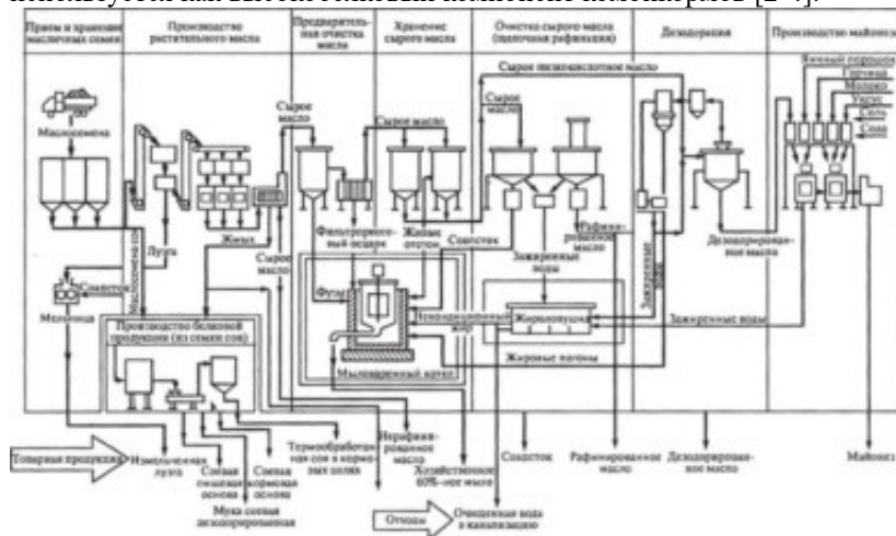
Рисунок 1 - Технология производства АО «ЭФКО»
