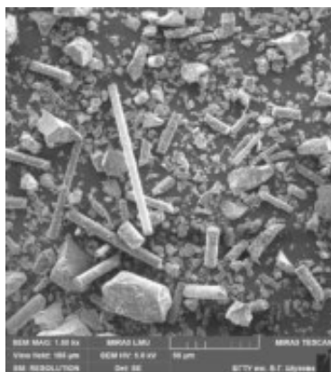
Рисунок 4 – Микрофототорграфии образцов ОТМ
