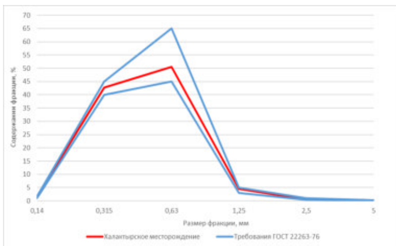
Рисунок 3 – Соотношение частиц различной фракции Халактырского песка относительно ГОСТ 22263-76
