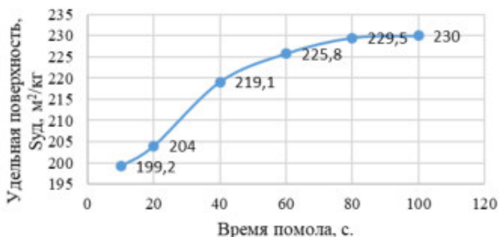
Рисунок 2 – Зависимость удельной поверхности ОТВ от времени помола
