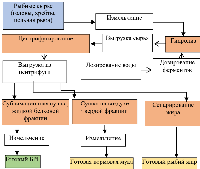
Рисунок 1 – Технологическая схема производства БРГ ферментативным методом
