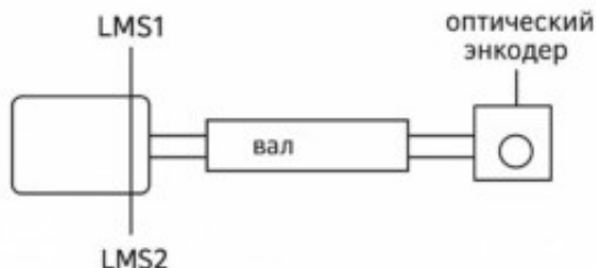
Рисунок 1 - Схема экспериментальной установки для измерения частоты вращения с двумя ДЛМ и оптическим энкодером в качестве эталона
