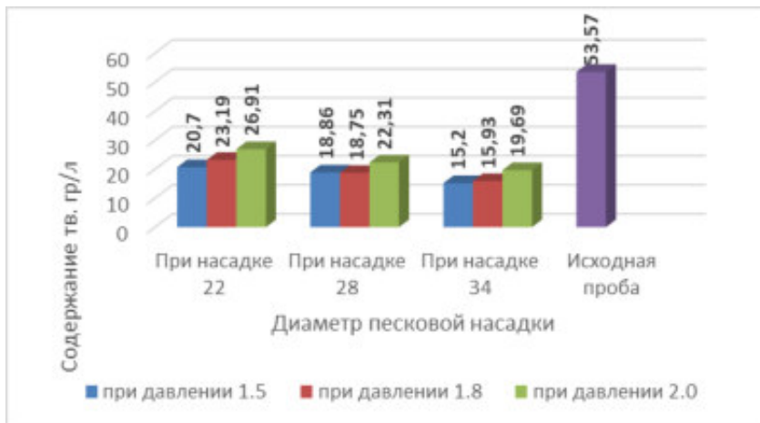
Рисунок 2.2. - Осветленный продукт (слив ГЦ)
