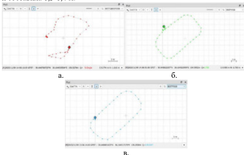
Рисунок 4 - Сравнение траекторий: а) Режим ГНСС, б) Режим ИНС, в) Гибридный режим ГНСС/ИНС*
