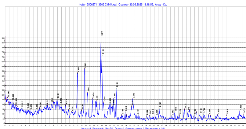
Рисунок 1 – Дифрактограмма Халактырского песка
