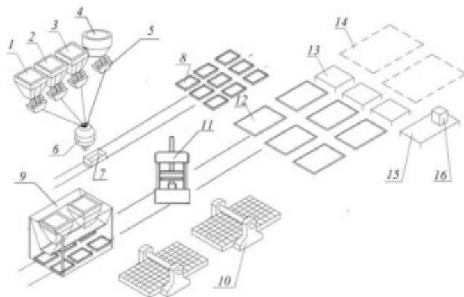
Рисунок 1 - Аппаратурная схема производства:
