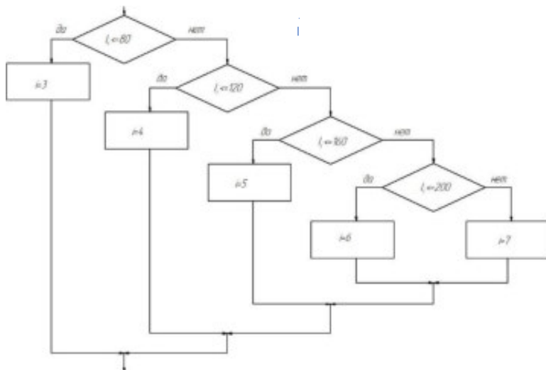
Рисунок 2 - Представление условий в виде блок-схемы для определения количества отверстий
