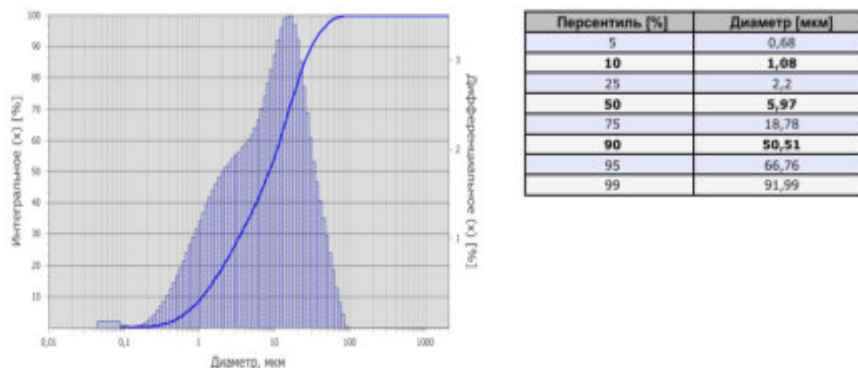
Рисунок 1 – Распределение по размерам и количество частиц тонкомолотого ОМ
