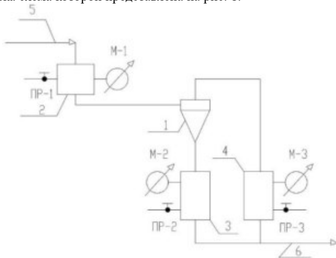
Рисунок 1 - Схема опытной установки
