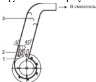
Рисунок 1 - Схема дробилки открытого типа с пневмосепаратором: 1 - решето; 2 - направляющие; 3 - отражатели [6].
