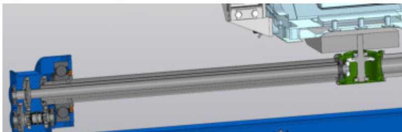
Рисунок 2 - Разрез механизма в составе portalной рамы
