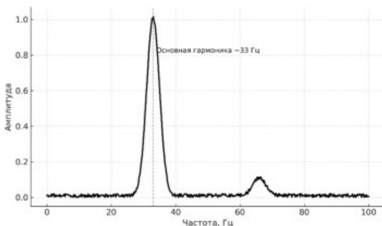
Рисунок 3 - Спектр взаимной зависимости при 2000 об/мин
