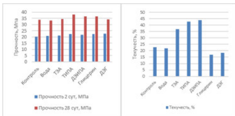
Рисунок 2 – Влияние добавок на прочность цемента
