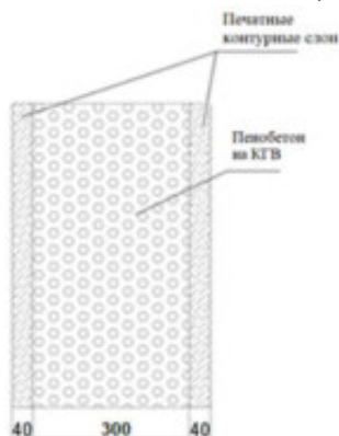
Рисунок 1 - Конструкция многослойной стены
