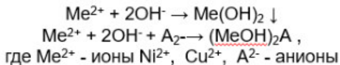
Рисунок 3 - Реагентный механизм очистки сточных вод термически модифицированной скорлупой лесного ореха.
