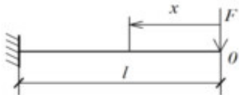
Рисунок 1 - Консоль
