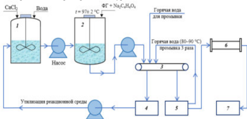
Рисунок 1 - Принципиальная схема пилотного испытания процесса превращения ФГ в \alpha -полугидрат гидротермальным методом [10]:
