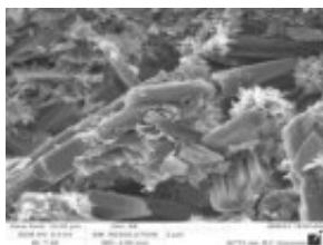
Рисунок 2 - Микроструктура затвердевшего КГВ с тонкомолотой минеральной добавкой ОМ
