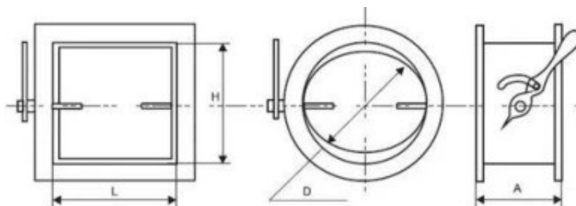
Рисунок 3 - Заслонка дискового типа с поворотным механизмом.
