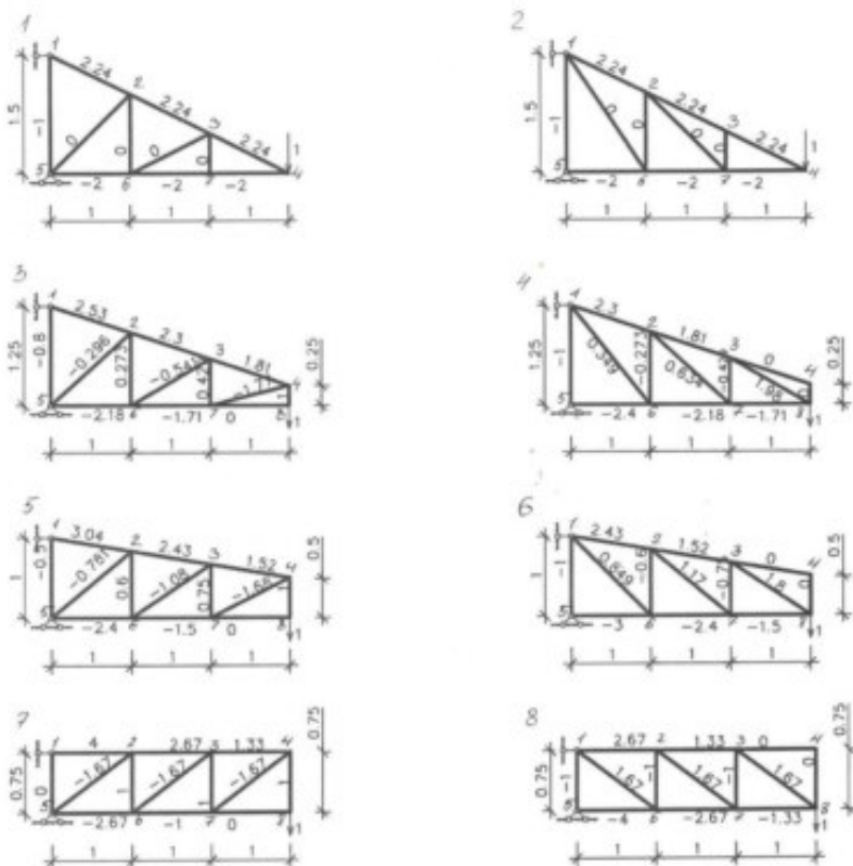
Рисунок 1 - Фермы 1-8 и продольные усилия ( N ) в стержнях от силы F = 1 Н
