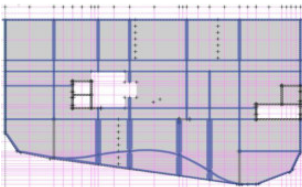
Рисунок 3 - Расчётная модель расположения диафрагм жёсткости и жёсткого диска перекрытия в монолитном каркасном здании (ETABS)
