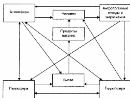
Рисунок 1 - Схема миграции загрязняющих веществ в окружающей среде
