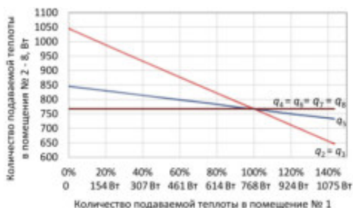
Рисунок 2 - Необходимое количество теплоты для поддержания в помещениях температуры 20°C при изменении количества теплоты, подаваемого в помещение № 1
