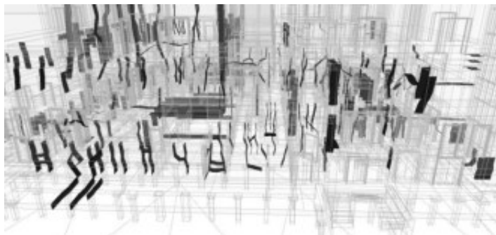
Рисунок 4 - Модели дефекта в цифровой модели здания для визуального анализа характера и динамики развития
