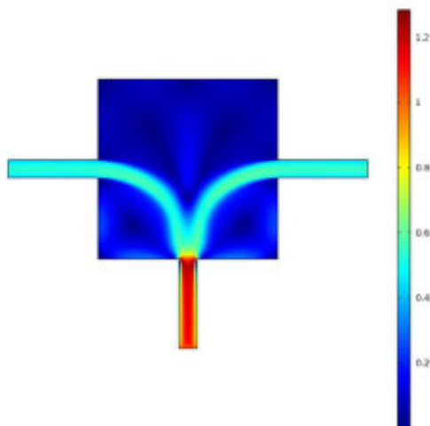
Рисунок 2 - Распределение скорости в области проектирования
