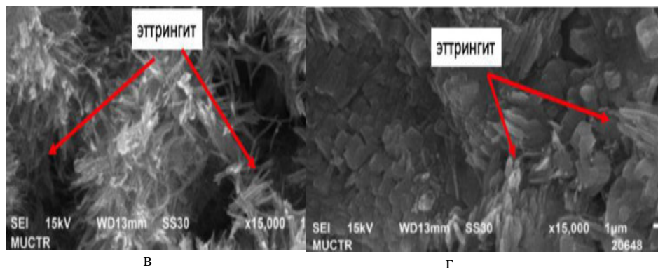
Рисунок 1 - Влияние вида сульфатированных клинкеров на структуру ПЦ, твердевшего 28 сут. при твердении морской воды Портландцемент: а – Г-5, б – С-2 (86% ПЦ + 7% САФК + 7% Гипс), в - С-3 (86% ПЦ + 7% САК + 7% Гипс), г -С-4 (86% ПЦ + 7% СФК + 7% Гипс). Увеличение x 15 000
