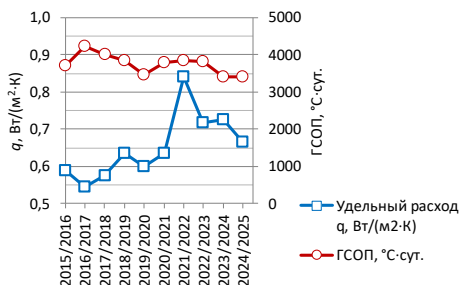
Рисунок 3 - Характеристики отопительных сезонов
