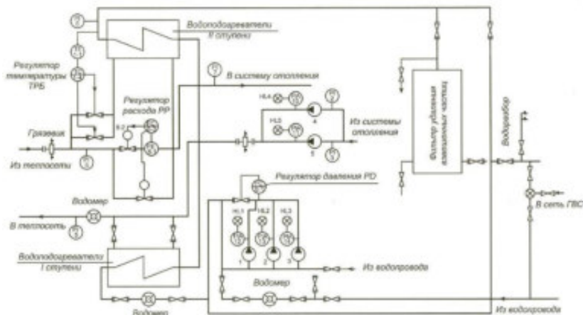
Рисунок 1 - Схема автоматизации тепловых сетей
