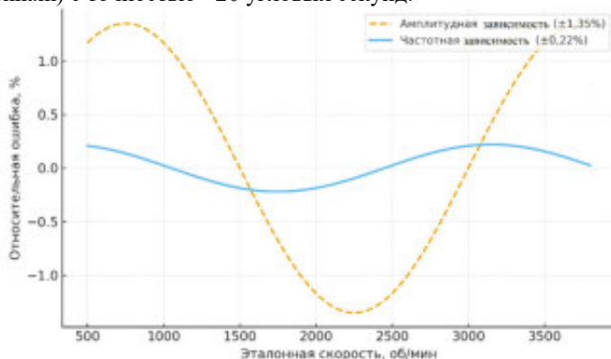
Рисунок 2 - График нелинейности двух методов измерения частоты вращения
