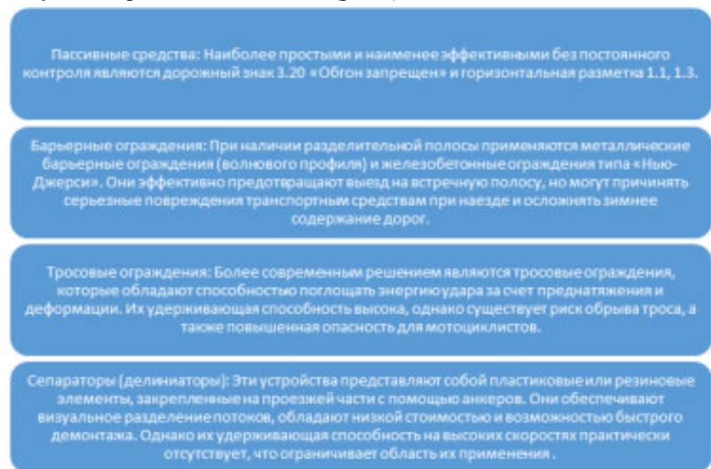
Рисунок 1 – Технические средства для разделения транспортных потоков
