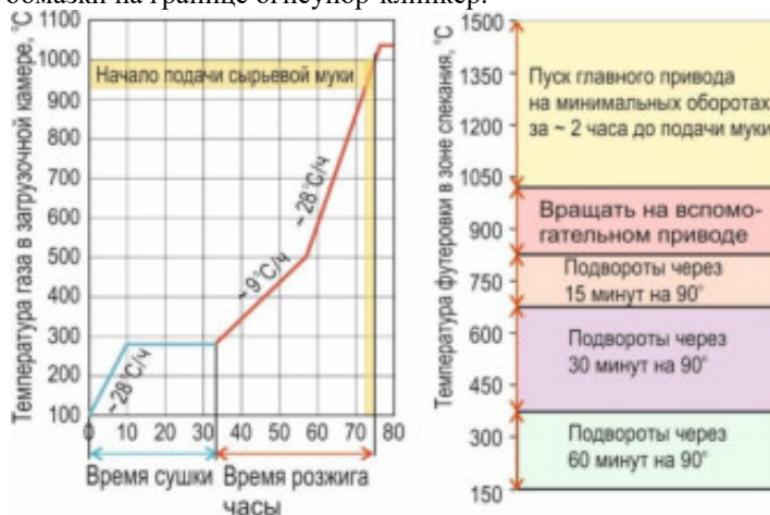
Рисунок 1 - Пример графика розжига при первичном пуске печи сухого способа [2]
