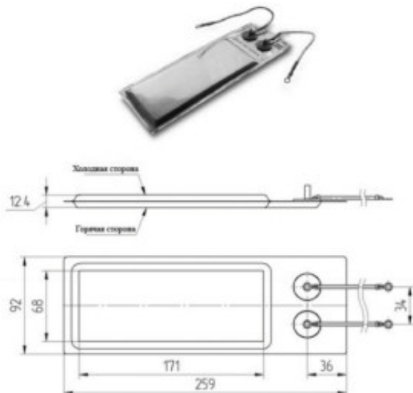
Рисунок 1 - Общий вид термоэлектрического модуля MARC-65
