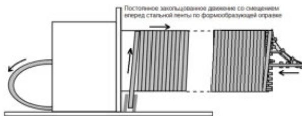
Рисунок 4 – Схема оправки машины непрерывной намотки
