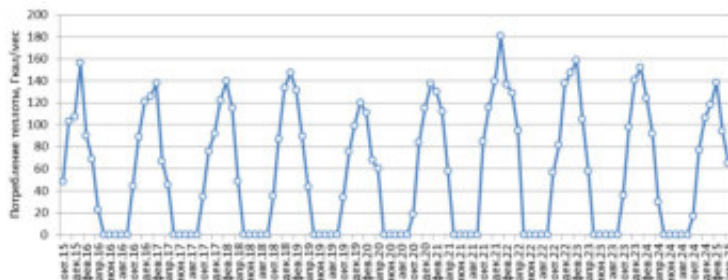
Рисунок 1 - Затраты теплоты на отопление
