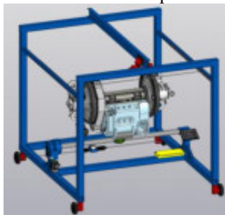
Рисунок 2 - Цифровая модель ПМПС
