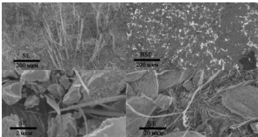
Рисунок 1. – Микрофотографии нановолокон хризотила с включенными микрочастицами ZrH_2 :
