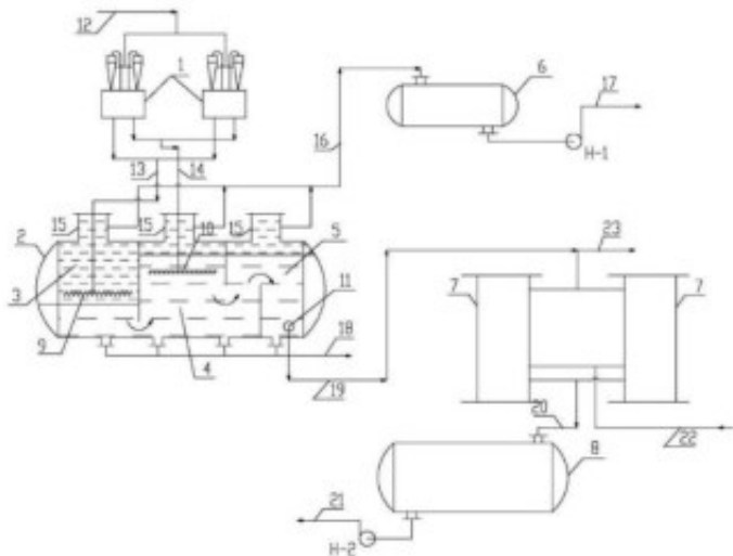
Рисунок 1 - Установка предварительного сброса с очисткой отделяемой пластовой воды.
