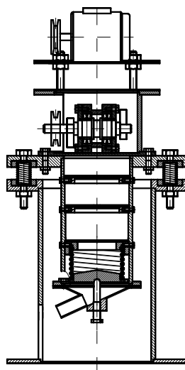
Рисунок 1 - Вибрационная мельница
