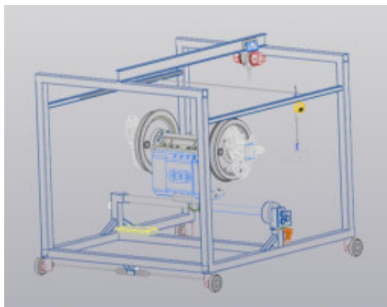
Рисунок 1 - Модель портала в APM FEM
