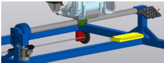
Рисунок 1 - Схема размещения оси и точек фиксации КМБ
