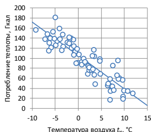
Рисунок 4 - Отопительная характеристика здания
