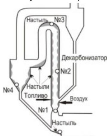
Рисунок 2 - Места образования настывлей в печах сухого способа производства
